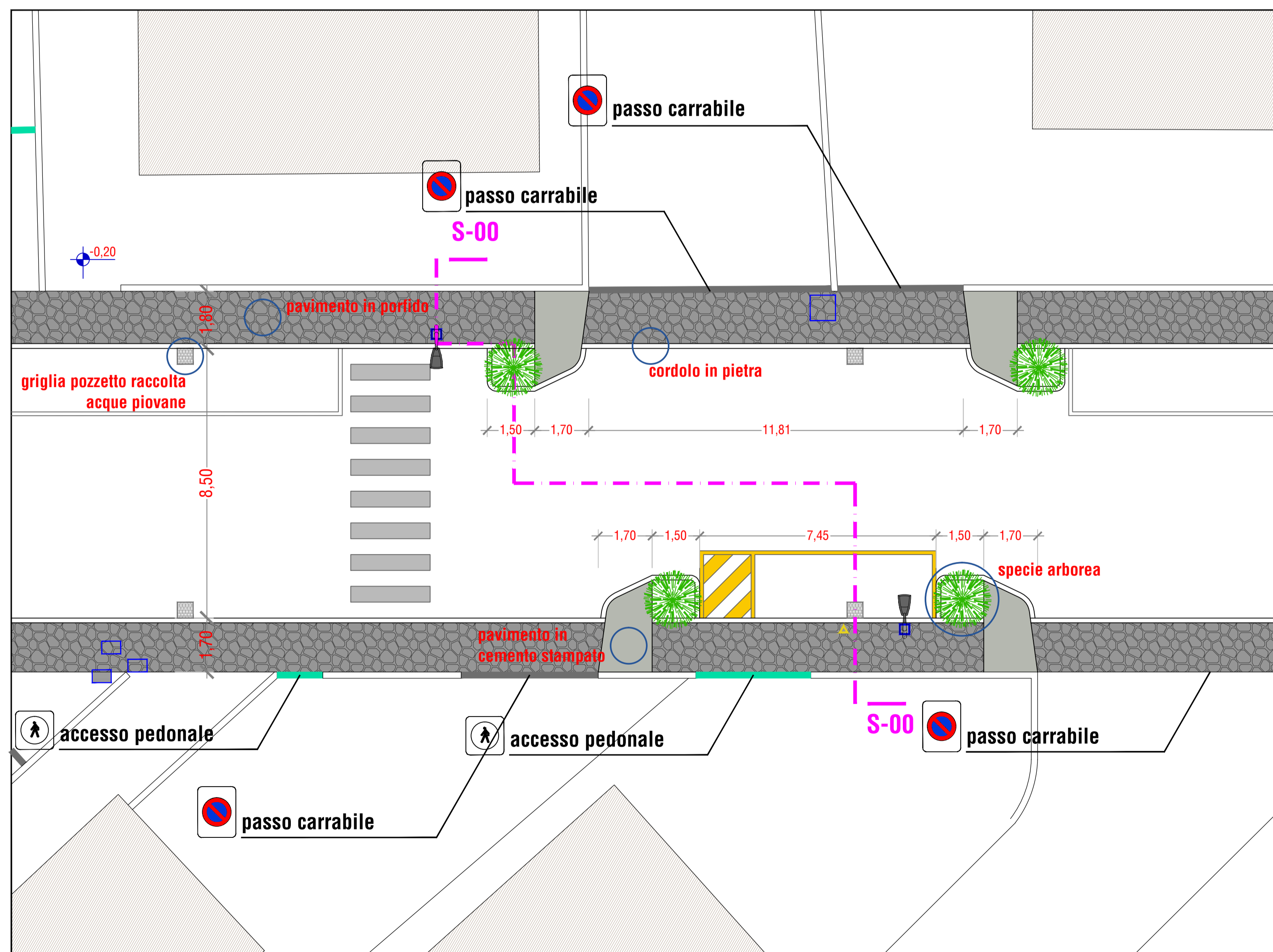
STRALCIO PLANIMETRIA STATO DI PROGETTO scala 1:100
