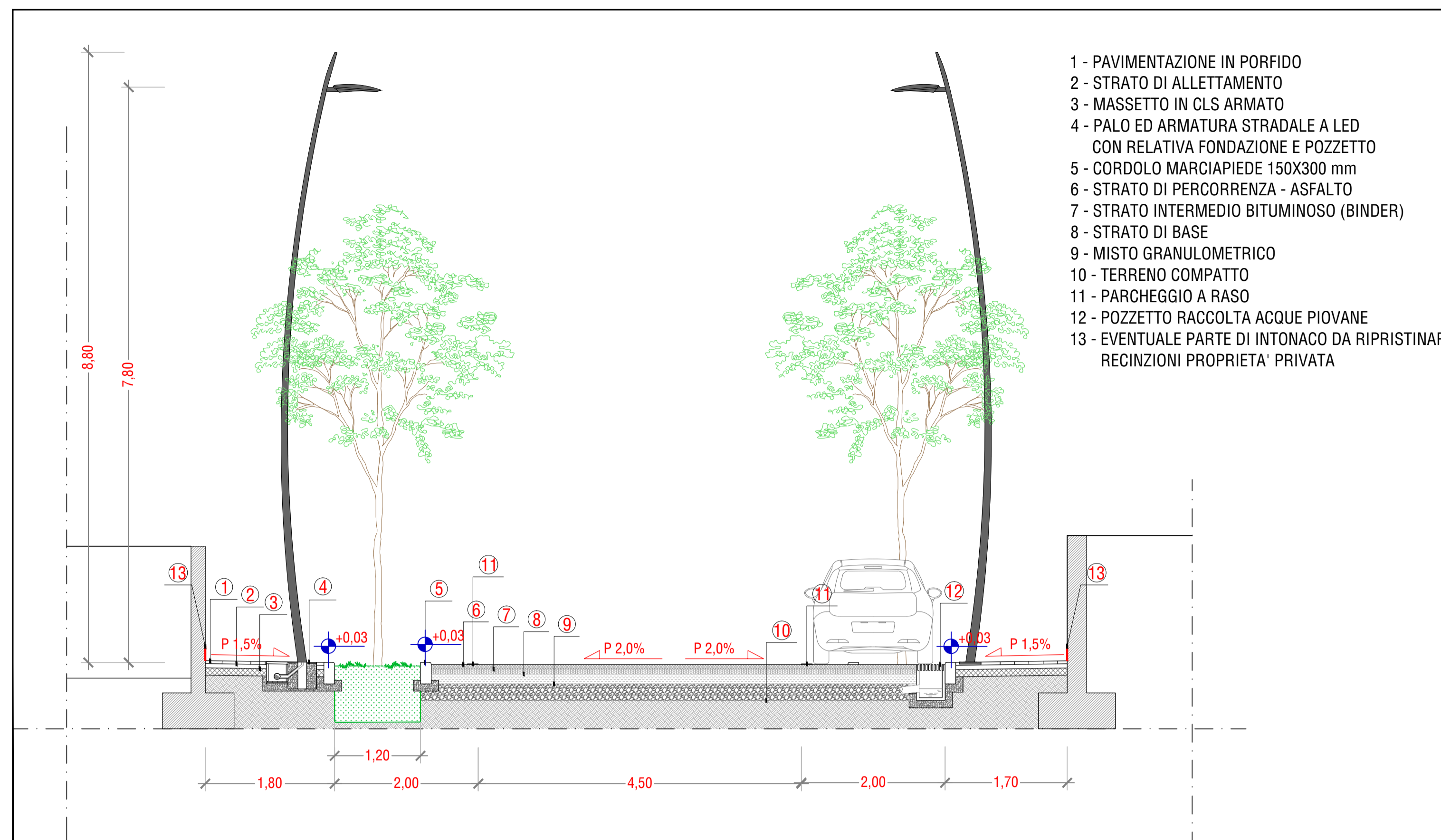
SEZIONE TIPO S-00 scala 1:50
