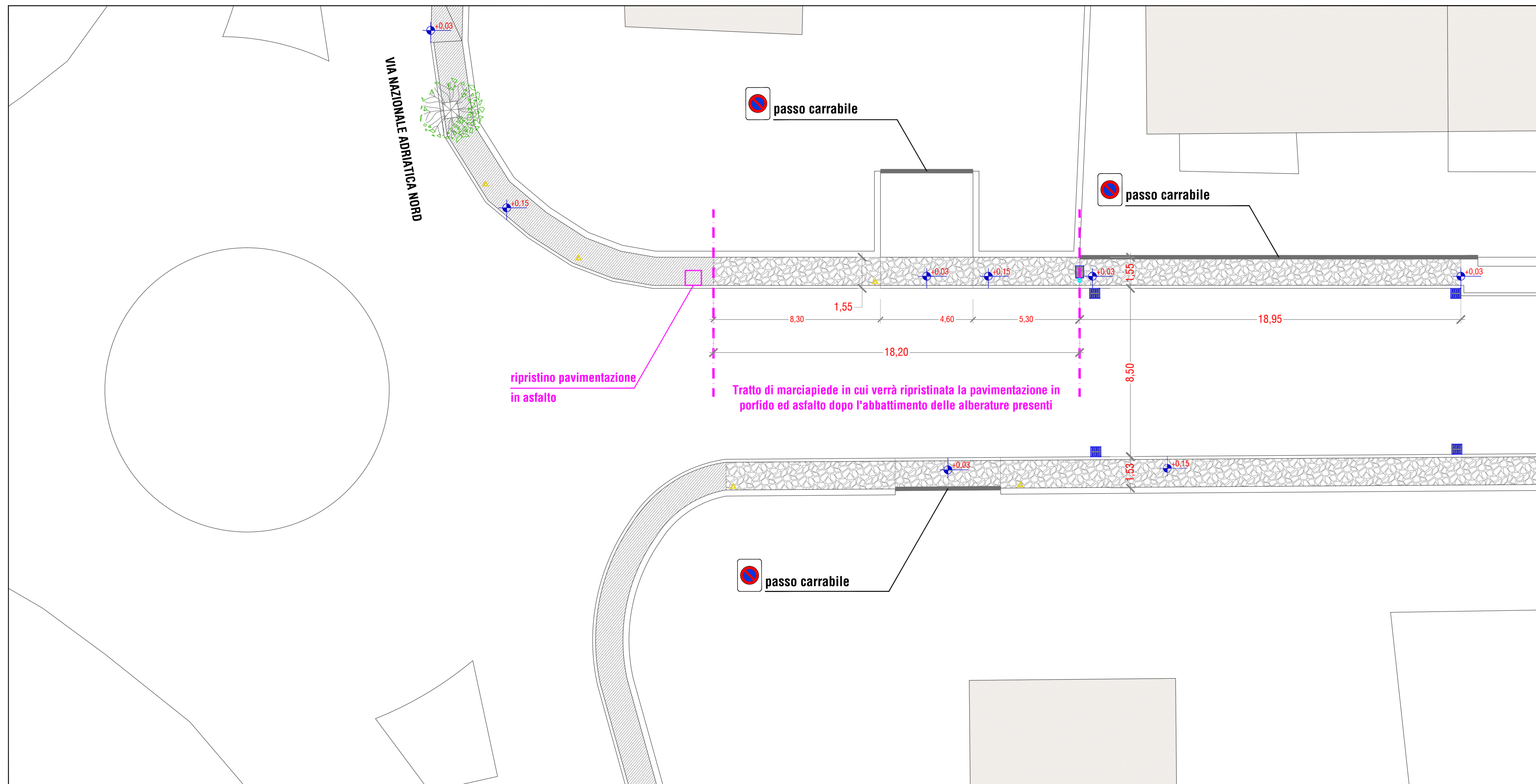
PLANIMETRIA STATO DI FATTO - Tratto compreso tra Via Nazionale Adriatica Nord e Via Fiume/Via delle Driadi scala 1:100
